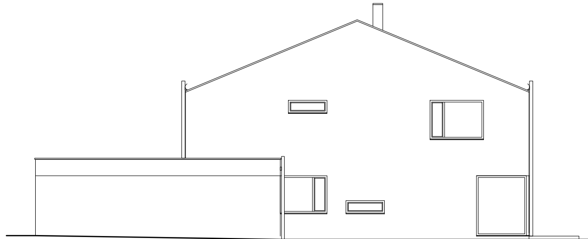
POHLED JIŽNÍ
