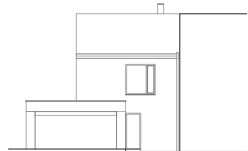
POHLED ZÁPADNÍ
