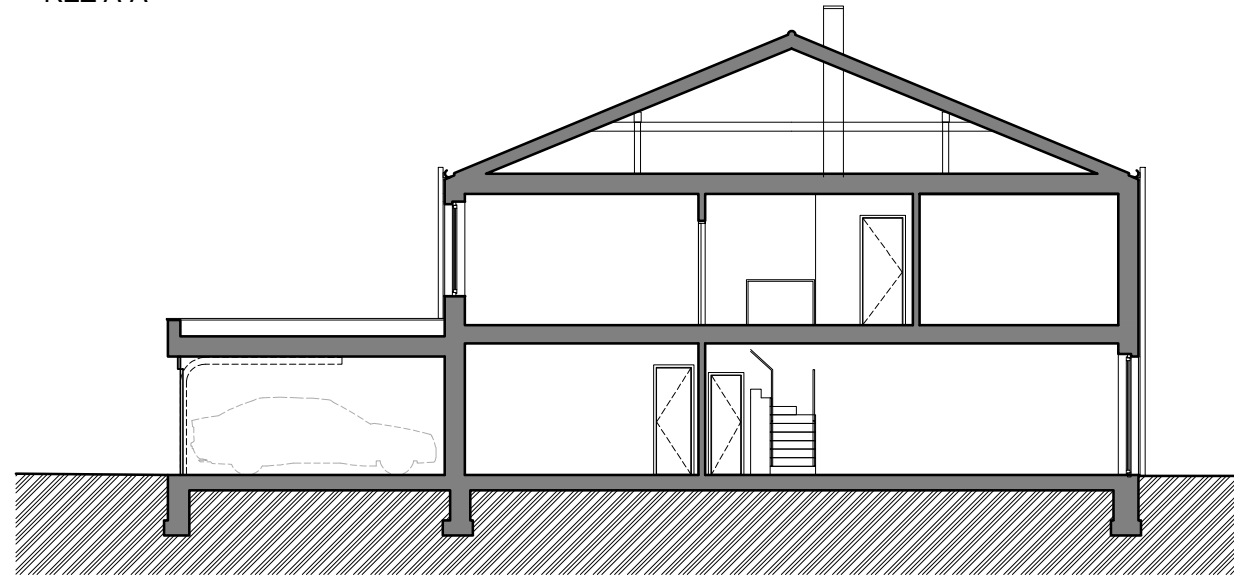
ŘEZ A-A'
