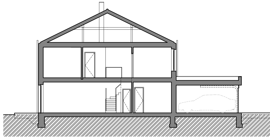
ŘEZ A-A'
