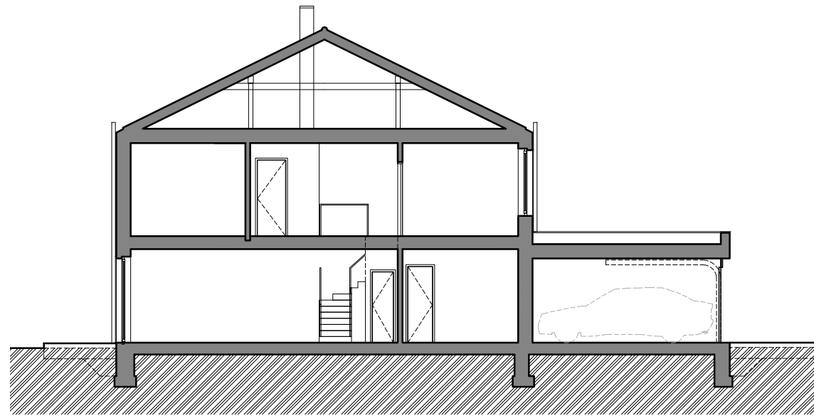
ŘEZ A-A'
