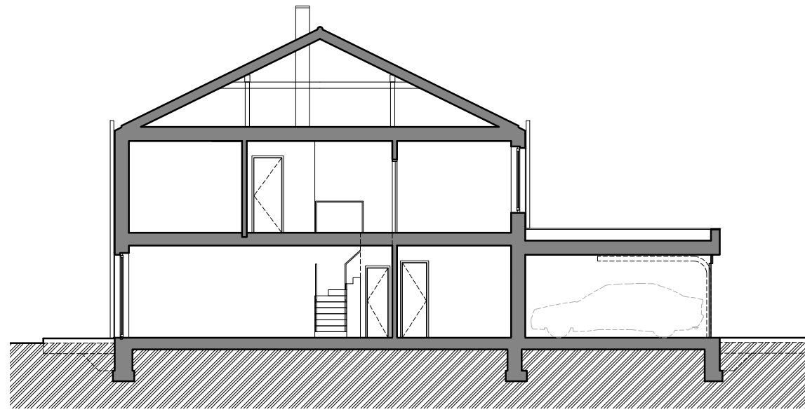
ŘEZ A-A'
