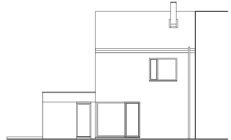
POHLED ZÁPADNÍ
