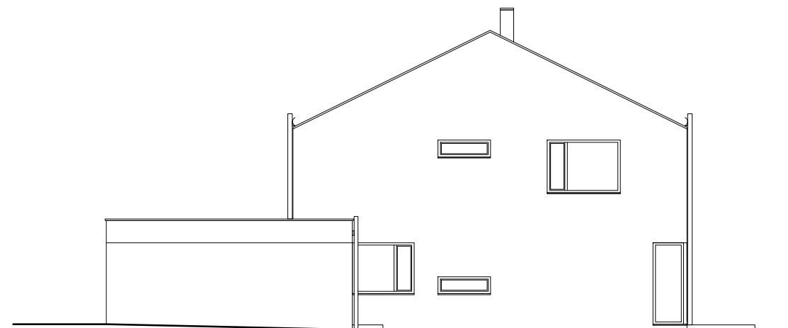
POHLED SEVERNÍ
