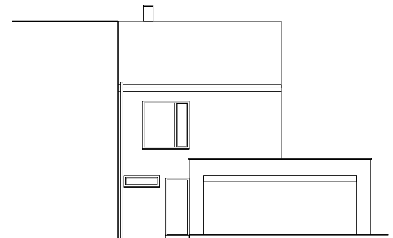
POHLED VÝCHODNÍ
