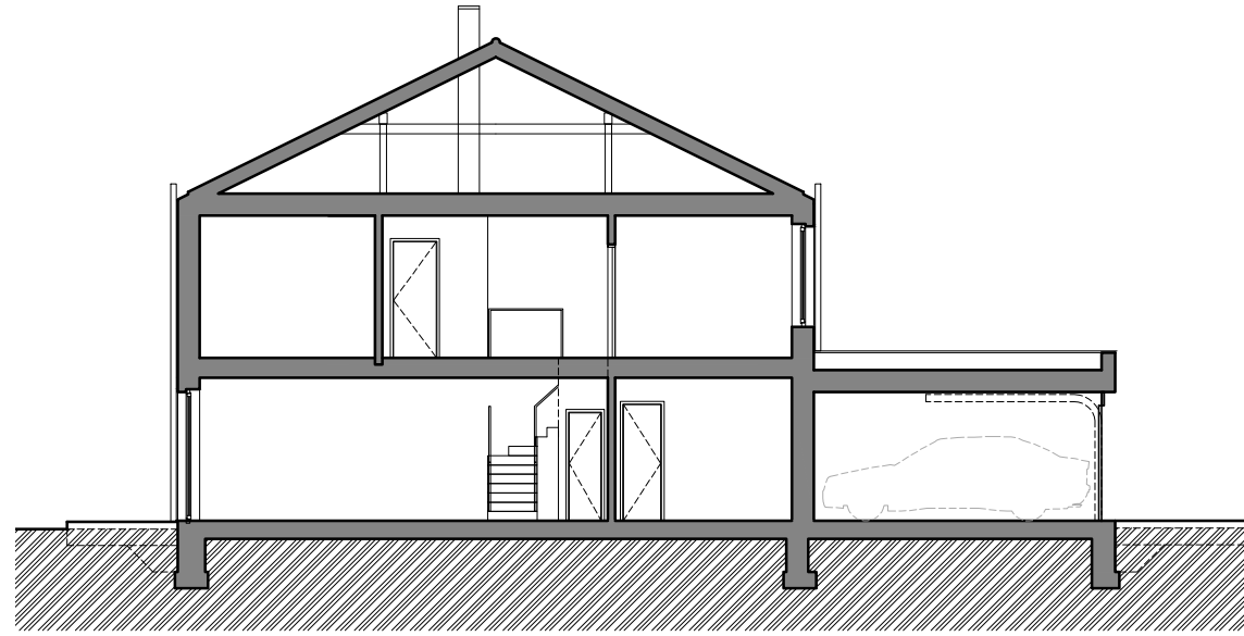
ŘEZ A-A'
