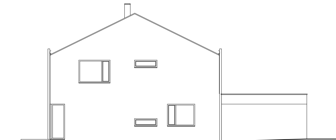
POHLED SEVERNÍ
