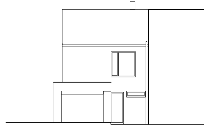
POHLED ZÁPADNÍ
