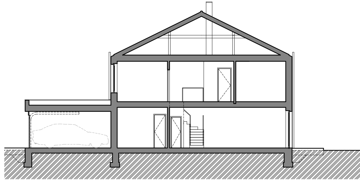
ŘEZ A-A'
