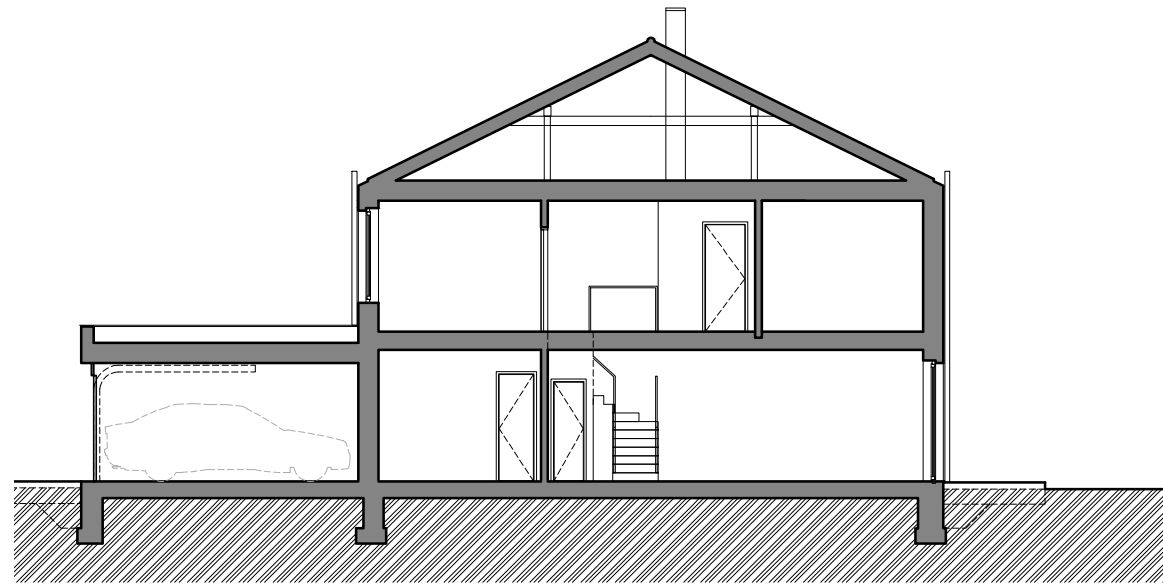
ŘEZ A-A'
