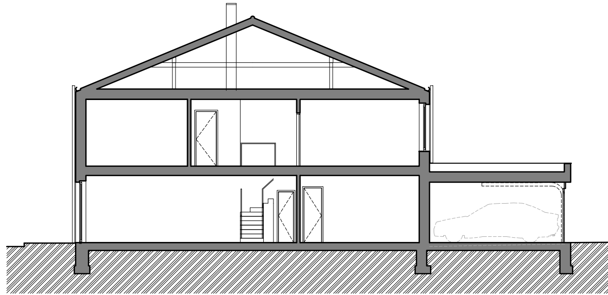
ŘEZ A-A'
