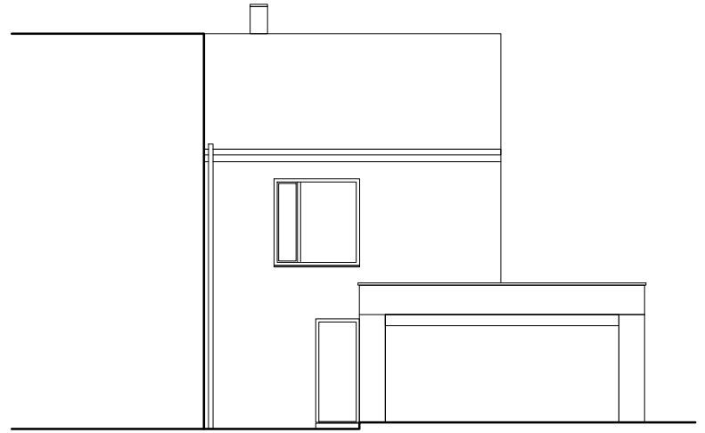
POHLED VÝCHODNÍ
