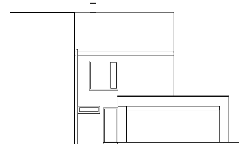
POHLED VÝCHODNÍ
