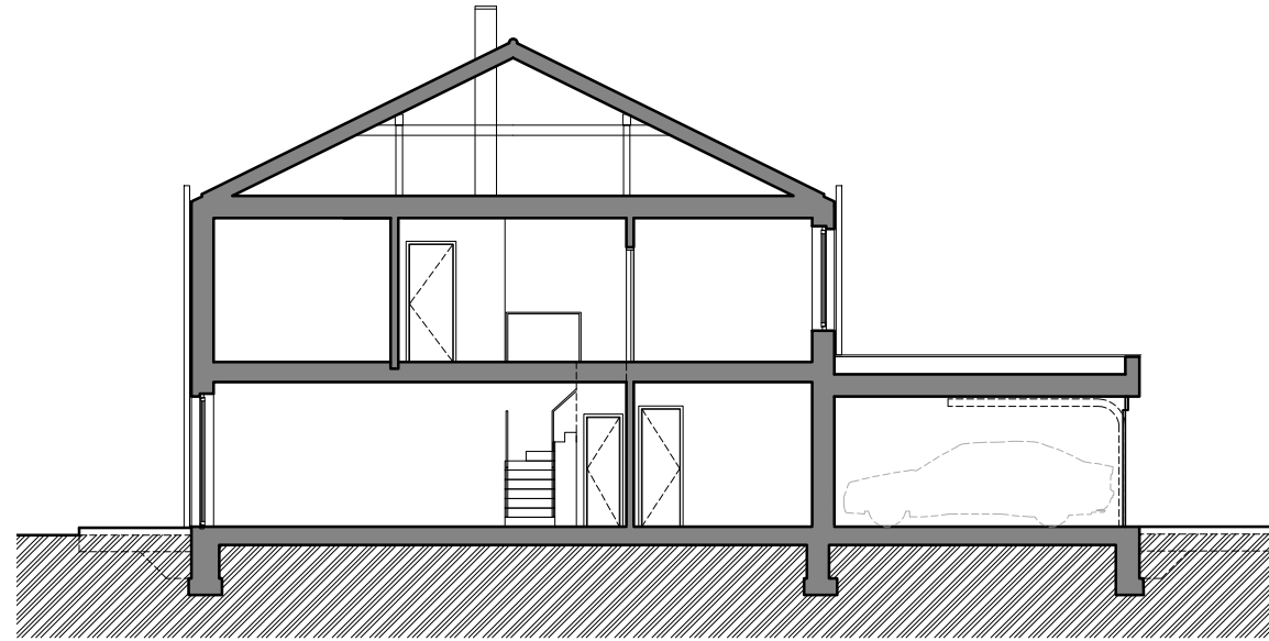
ŘEZ A-A'
